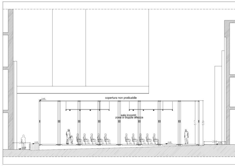
PROSPETTO EST /SEZIONE LONGITUDINALE - SCHEMA INDICATIVO
