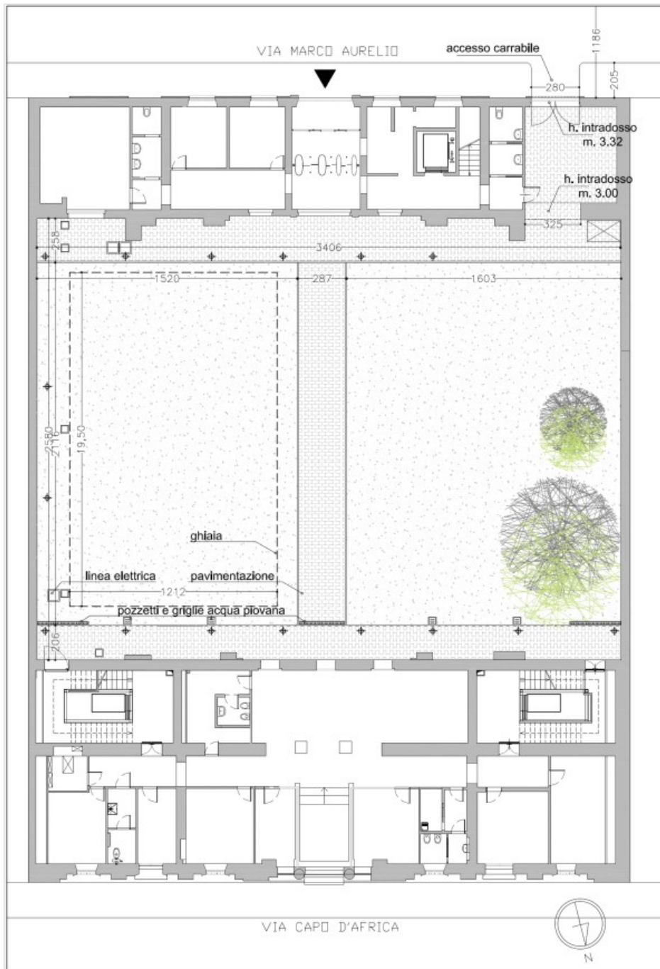
PIANTA 1 - STATO ATTUALE
