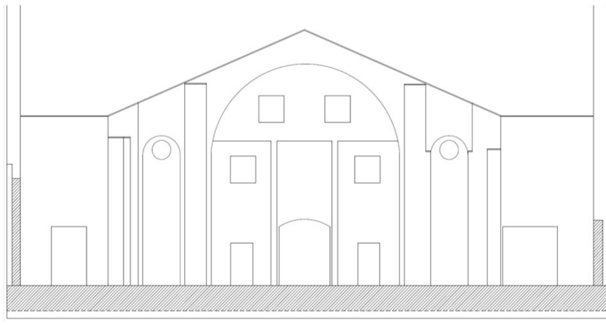
PROSPETTO SUD - STATO ATTUALE
