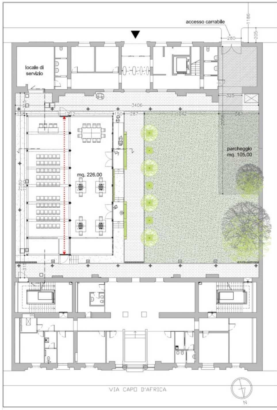
PIANTA 2 - SCHEMA INDICATIVO
